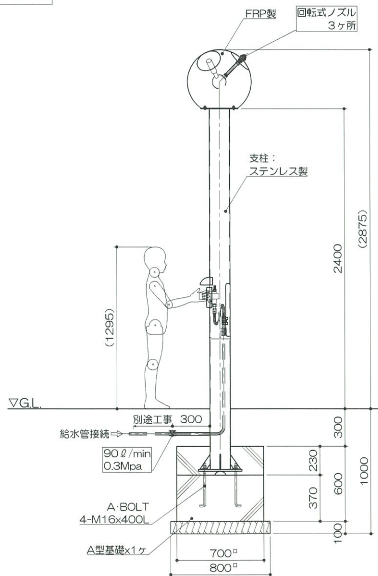
立面図 S= 1 : 30
