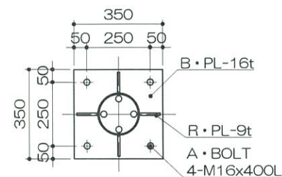
アンカープラン S= 1 : 20
