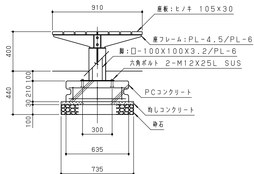
側面図 S = 1/20
