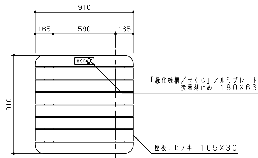
平面図 S = 1/20
