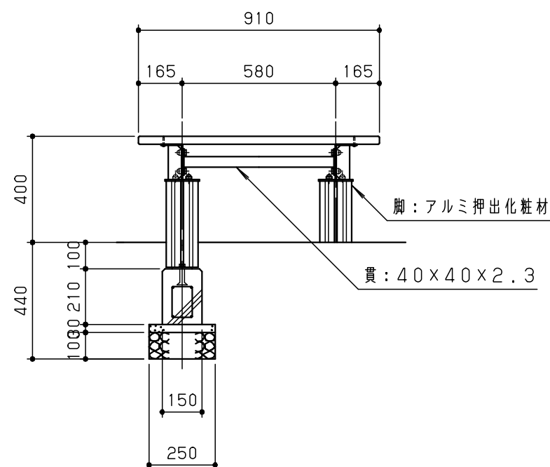
正面図 S = 1/20
