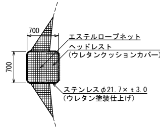
ハンモックシートW (ヘッドレスト付き) 展開図
