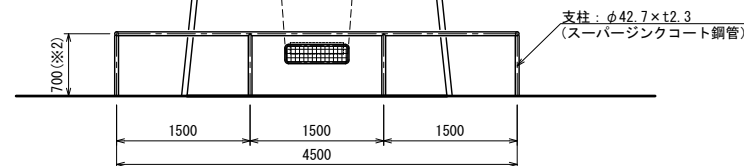
境界柵立面図
