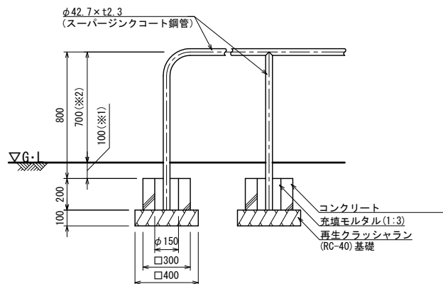
境界柵詳細図
