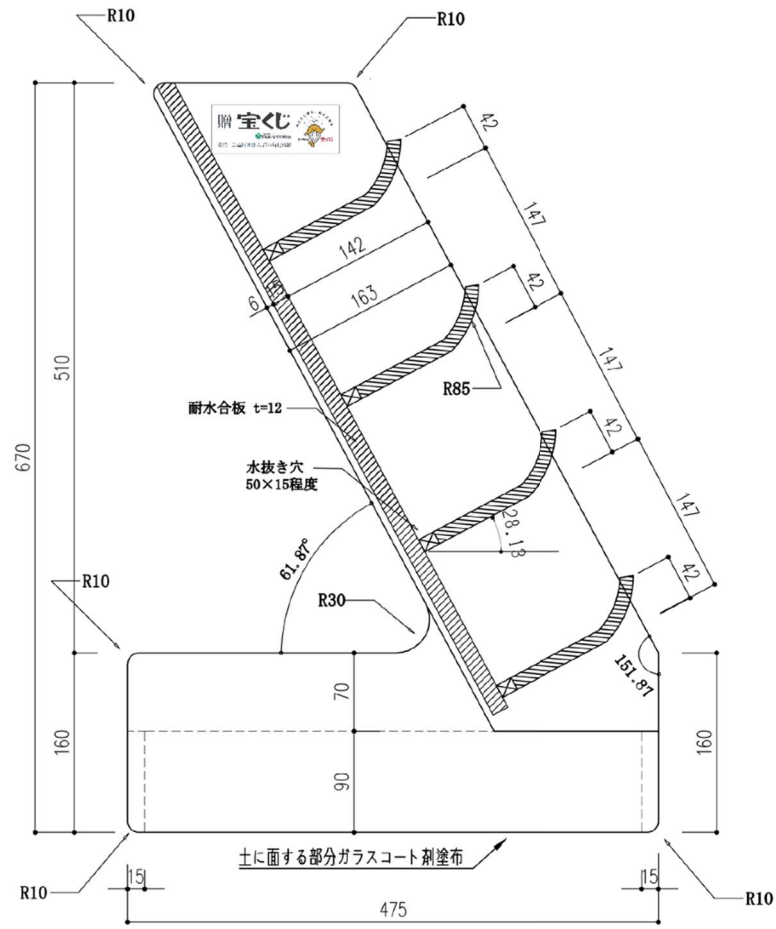
A-A' 断面図
