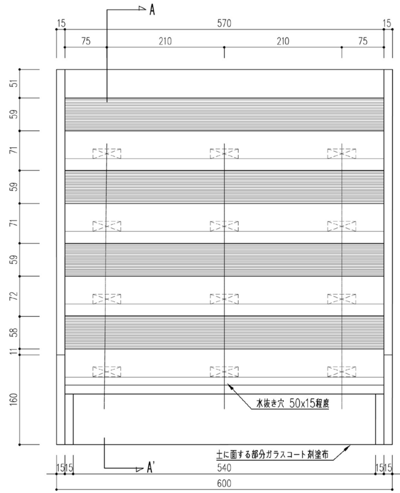
正面図
