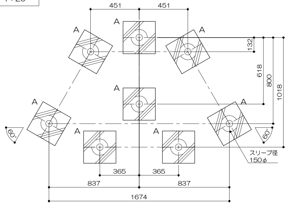
基礎平面図 S= 1 : 20
