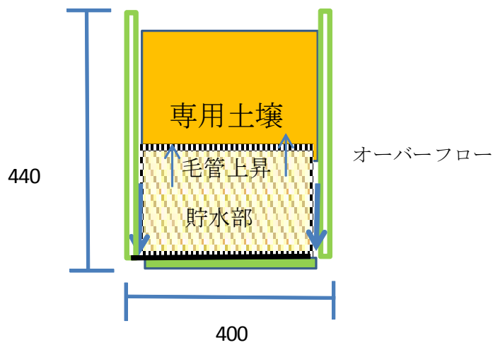
図2-縦方向から見た図
