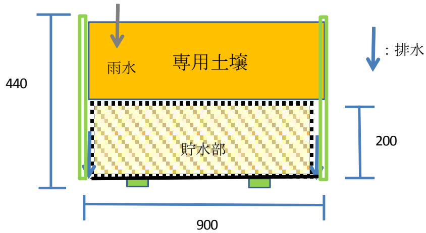
図1-横から見た図
