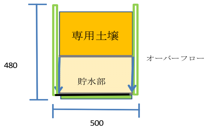
図2・縦方向から見た図
