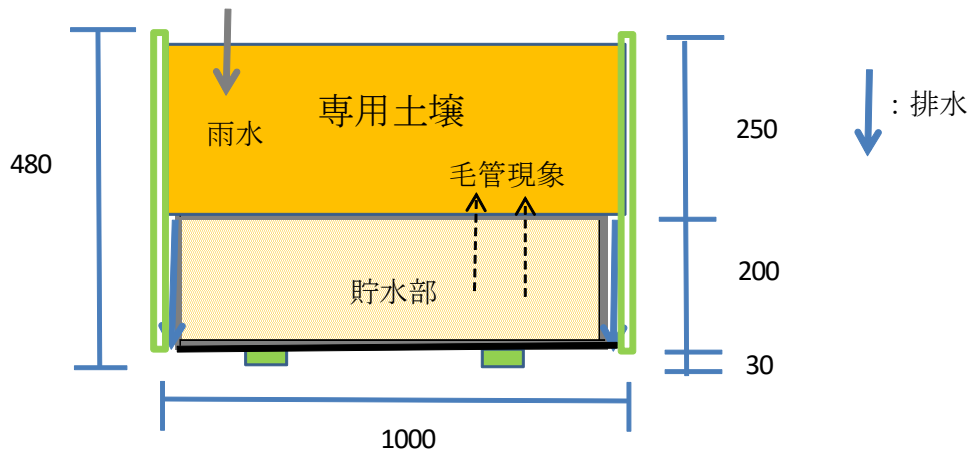
図1・横から見た図
